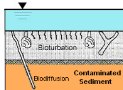
THIN CAP
